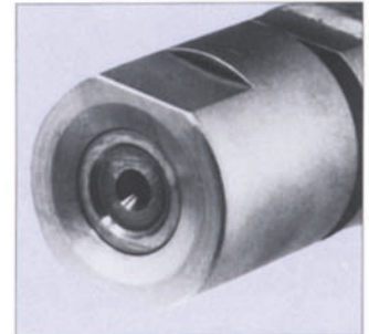
Spillback nozzle lance
